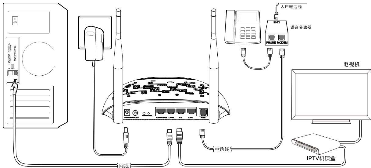
图 3 ADSL 宽带
